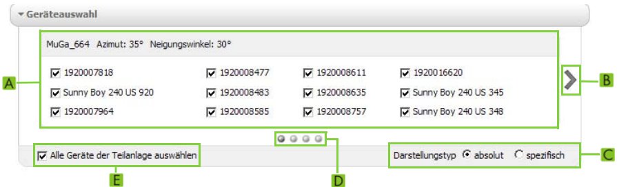
Abbildung 5: Aufbau des Einstellbereichs auf der Seite Wechselrichter
